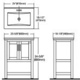
Basin: 610×470mm Cabinet: 600×460×880mm
