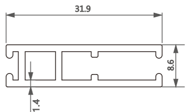
型号/Item No.-190718 米重/Weight-0.311kg/m
