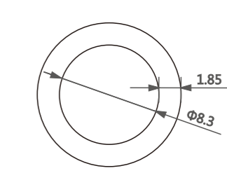
型号/Item No.-6110446 米重/Weight-0.16kg/m
