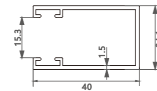
型号/Item No.-0901583 米重/Weight-0.466kg/m
