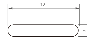
型号/Item No.-920010 米重/Weight-0.063kg/m
