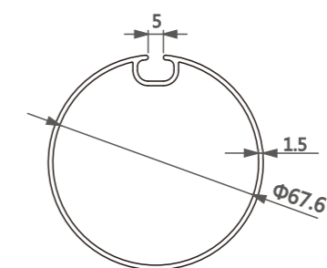
型号/Item No.-1118197 米重/Weight-0.970kg/m
