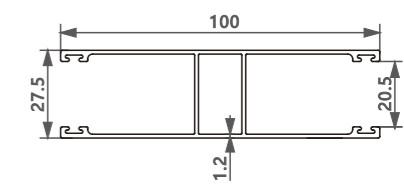
型号/Item No.-79081016-1.2 米重/Weight-0.945kg/m
