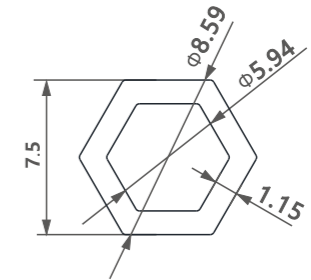
型号/Item No.-13031775 米重/Weight-0.069kg/m
