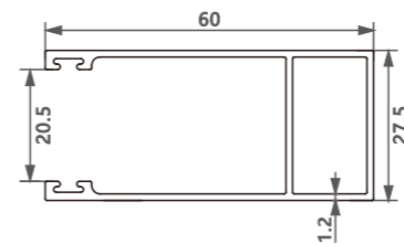
型号/Item No.-79081015-1.2 米重/Weight-0.62kg/m
