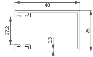
型号/Item No.-0901586 米重/Weight-0.424kg/m
